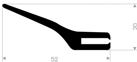
211.09.175 EPDM 65° Shore zwart rollengte 50 meter
