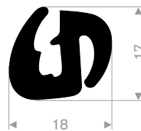
212.00.088 EPDM 70° Shore zwart rollengte 30 meter
