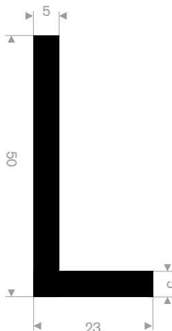
216.55.023 EPDM 60° Shore zwart rollengte 50 meter
