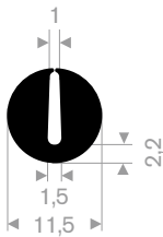
211.00.175 EPDM 70° Shore zwart rollengte 100 meter
