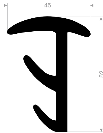
216.05.760 EPDM 70° Shore zwart rollengte 25 meter
