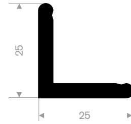
216.52.525 EPDM 60° Shore zwart rollengte 25 meter
