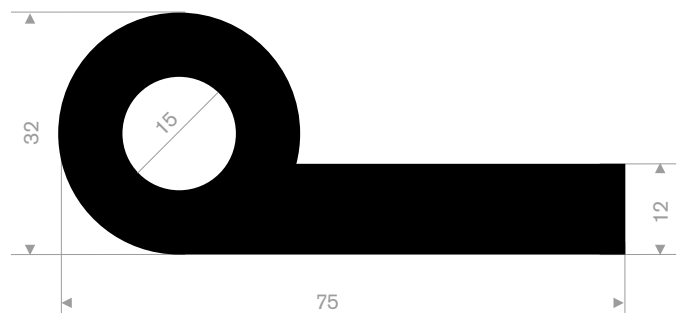
214.00.866 EPDM 70° Shore zwart rollengte 20 meter
