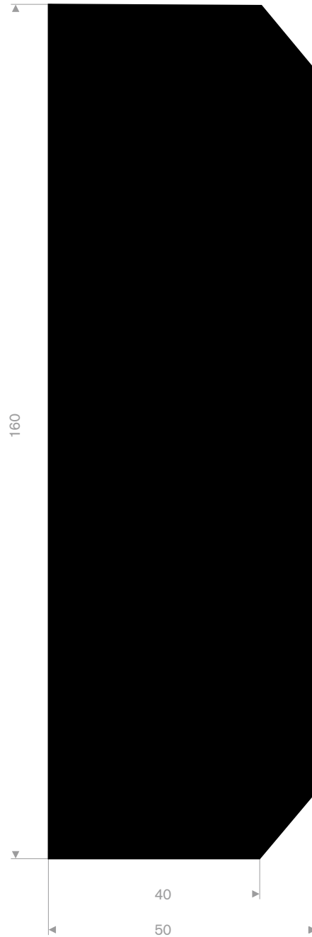
215.01.200 EPDM 70° Shore zwart rollengte 10 meter
