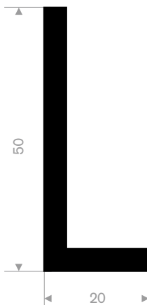
216.55.020 EPDM 70° Shore zwart rollengte 25 meter
